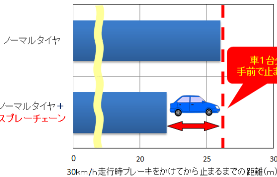
圧雪路制動試験
